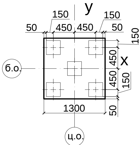
Рис. 12. Конструирование ростверка
