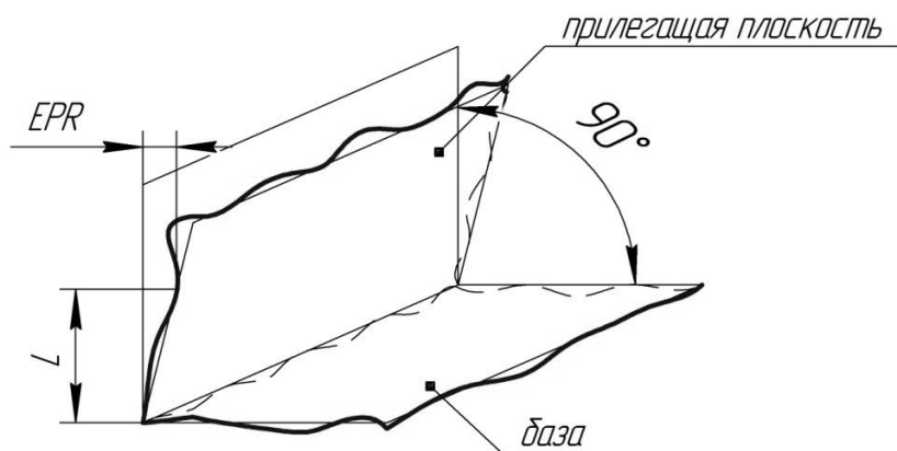
Рис.5. Отклонение от перпендикулярности плоскостей
