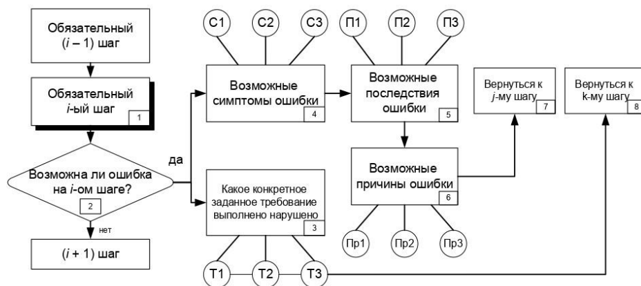
Рис. 1. Фрагмент блок-схемы самоконтроля возможных ошибок
