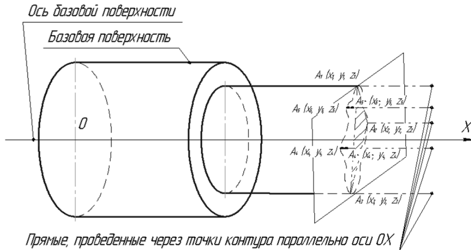
Рис. 3. Определение положения в пространстве плоскостей относительно контролируемой детали
