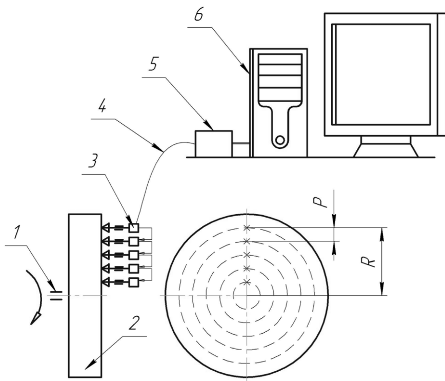
Рис. 6. Введение дополнительных позиций датчика
