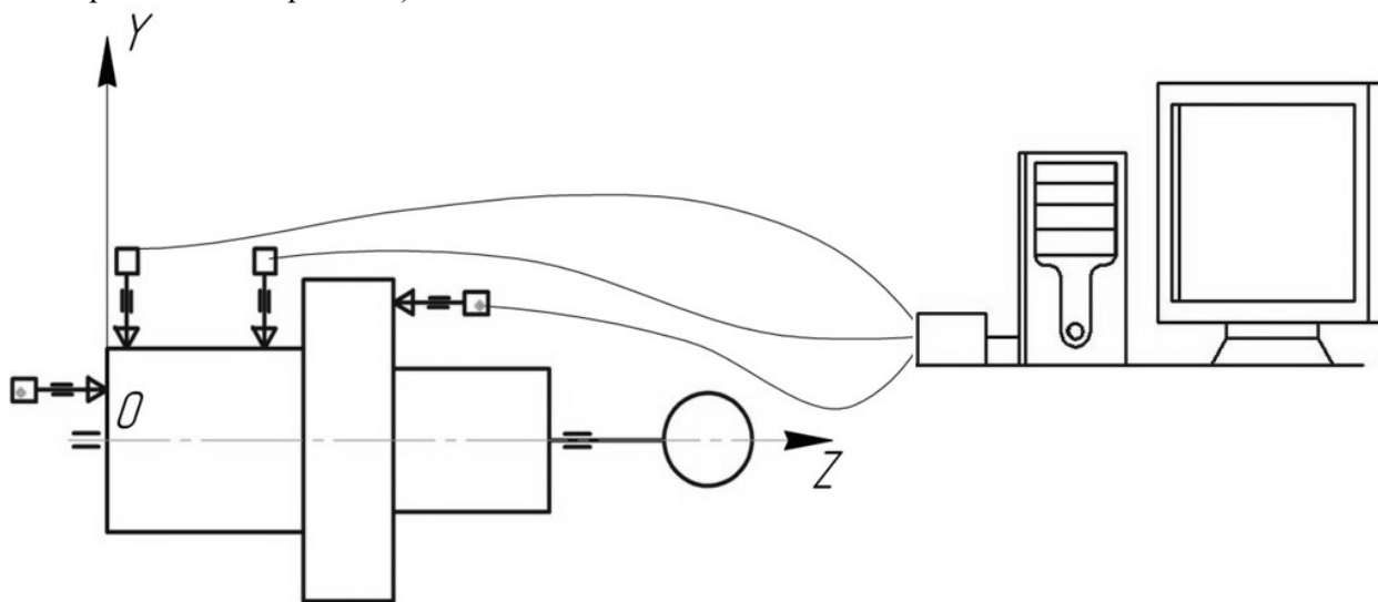
Рис. 1. Схема сбора координат точек при определении отклонения от плоскостности, перпендикулярности, параллельности, торцевого биения
