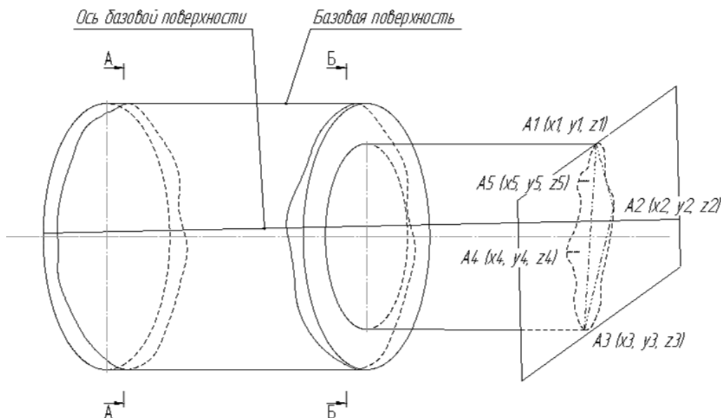
Рис. 2. Определение оси базовой поверхности, прилегающей плоскости
