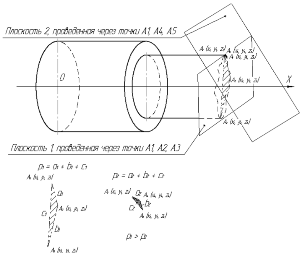
Рис. 4. Выбор прилегающей плоскости из множества по размеру базы Угол \psi между прямой и плоскостью определяется по формуле [9]:
