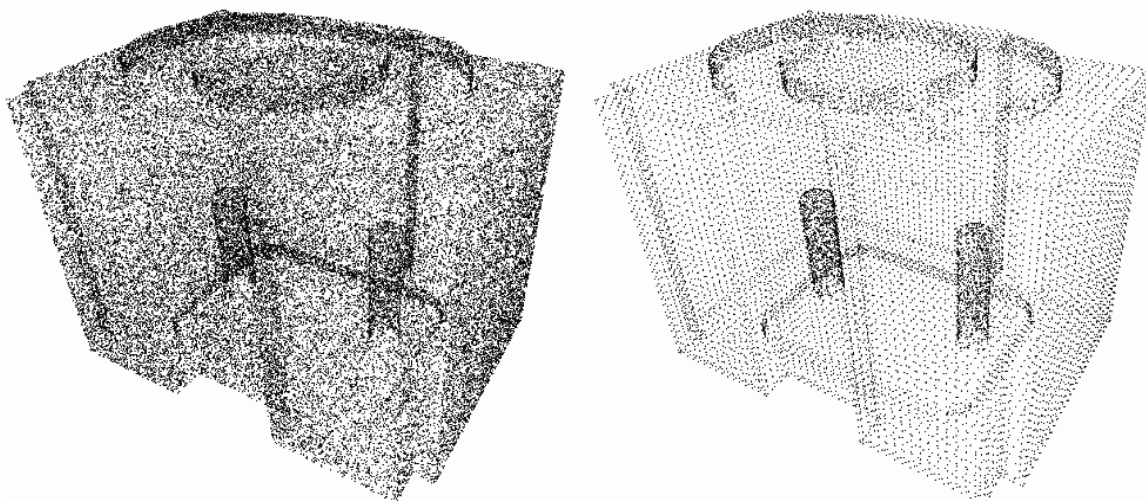
Рис. 9. Облако точек, полученное в результате сканирования детали в ходе реверсивного инжиниринга
