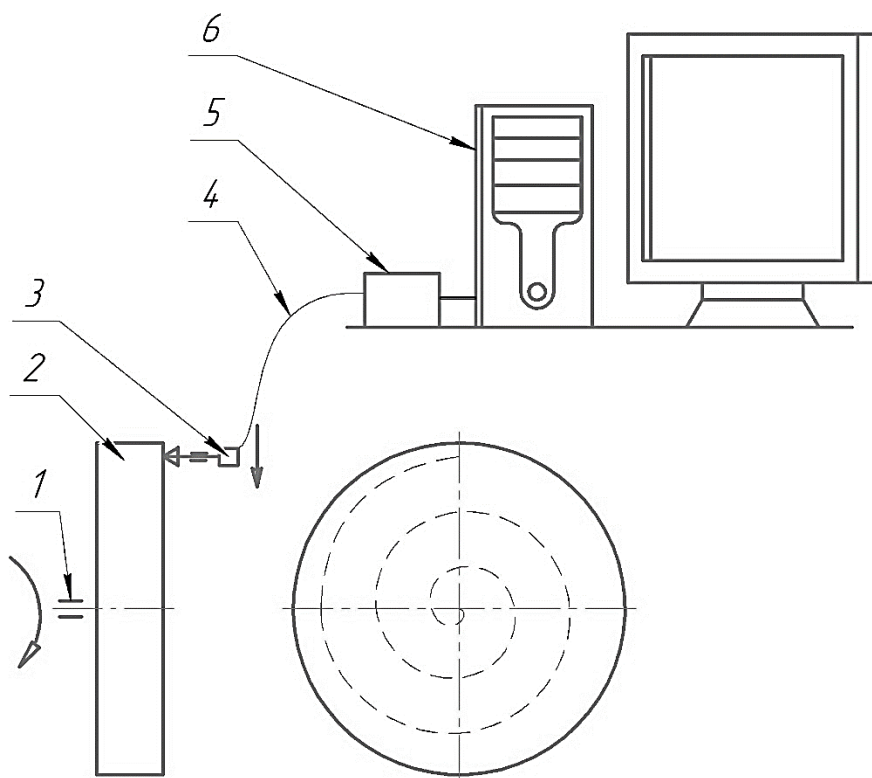
Рис. 7. Траектория сбора массива координат точек при одновременном вращении детали и перемещении датчика к оси
